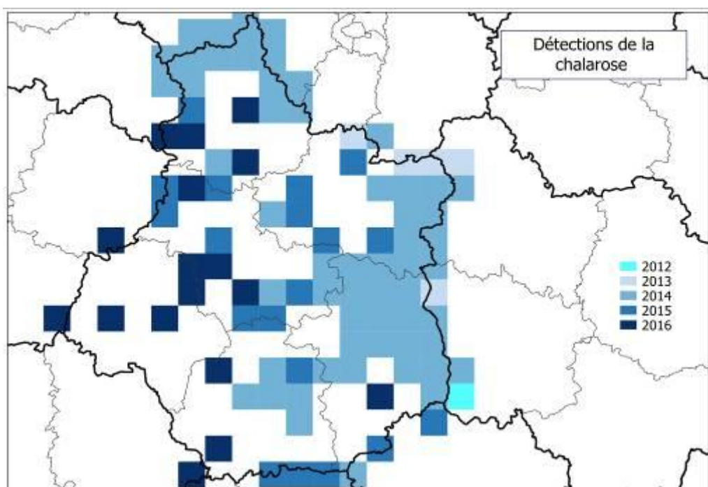
△ Fig. 13 – Evolution temporelle de la présence de la chalarose
