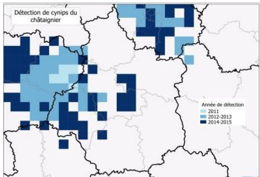
△ Fig. 12 – Carte de présence du cynips du châtaignier
