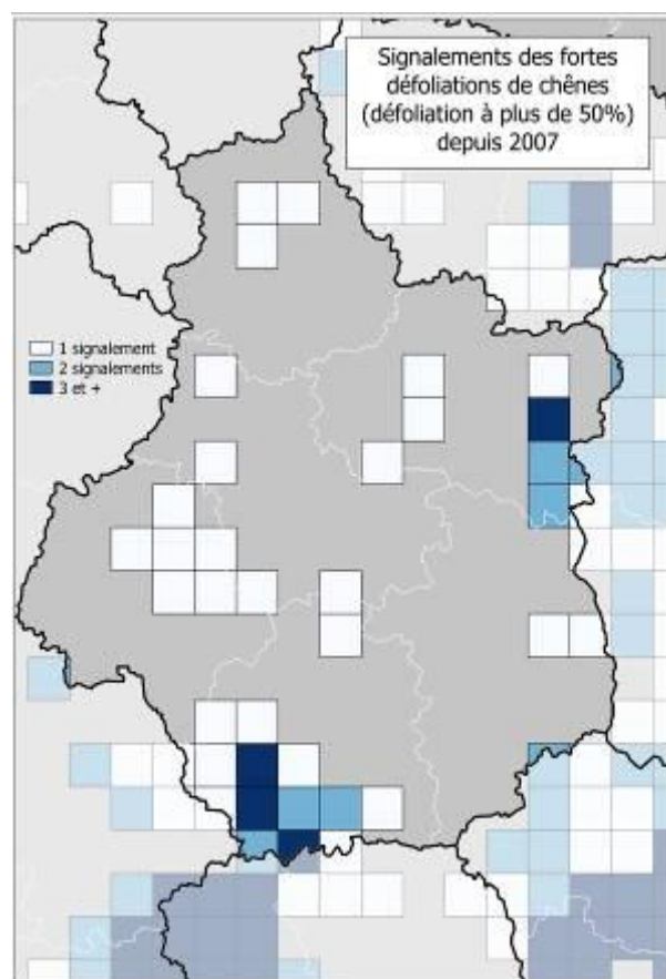
△ Fig. 8 - Signalement des chênes défoliés à plus de 50 % depuis 2007
