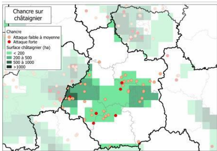
△ Fig. 10 – Signalement de la présence du chancre sur châtaignier
